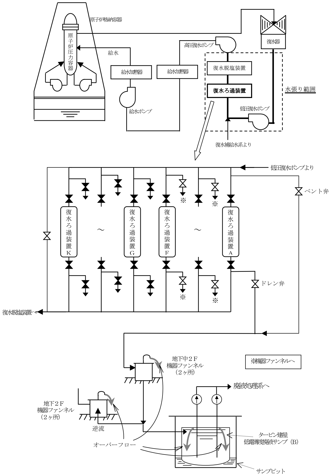
1号機 系統概略図
