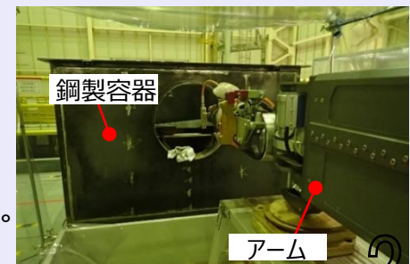
<試験装置外観>
