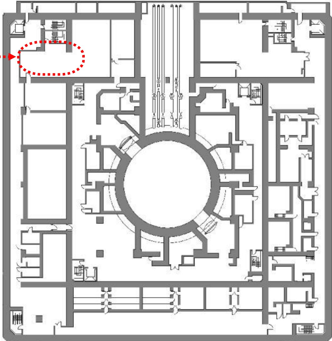
柏崎刈羽原子力発電所5号機 原子炉建屋 地下1階
