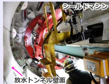
シールドマシン内部で後方から前方部を撮影 <シールドマシン掘進作業の状況>
