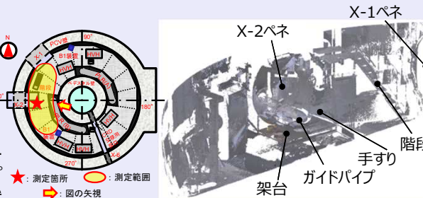
<X-2ベネレーンション周辺のレーザスキャン測定結果>
